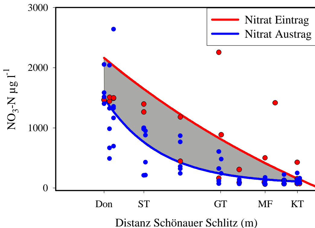
Abb. 10: Zusammenhang Distanz zum Schönauer Schlitze und Nitratkonzentration bei Hochwasser, differenziert in ein- und ausströmende Situationen. Don: Donau, Abkürzungen siehe Abb. 1.
