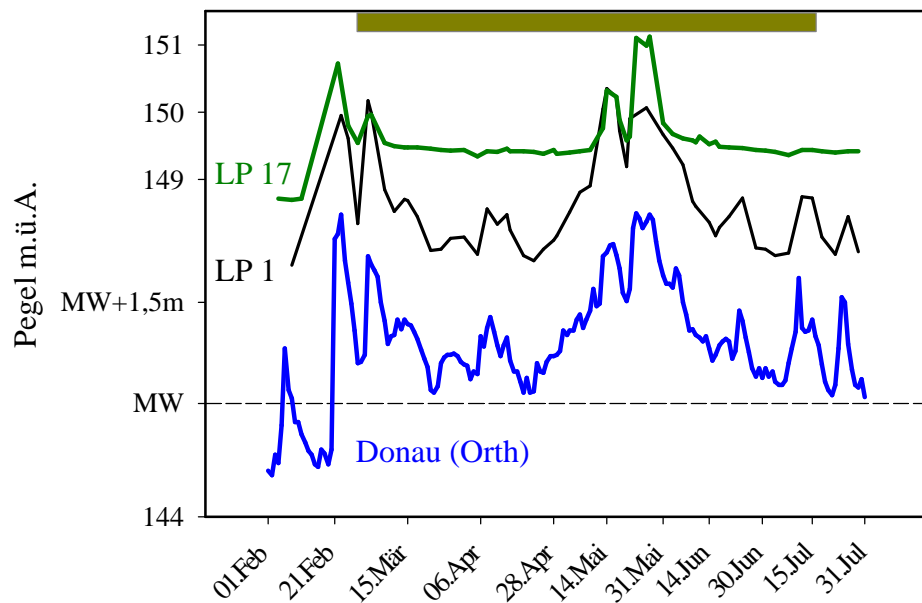
Abb. 3: Pegel Orth (Donau), Pegeldata innerhalb des Ausystems, Standorte der Lattenpegel lt. Abb. 2. MW: Mittelwasser laut KWD 1996 (WSD 1998). Balken deutet Untersuchungsperiode an.
