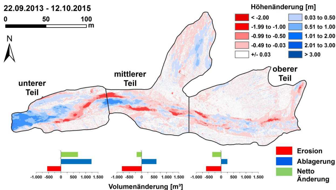
Figure A.2.9: Sedimentverlagerung im Gsenggraben – rote Farben zeigen Erosion, blaue Farben Ablagerung (Grafik aus: Rascher und Sass, 2017, verändert).
