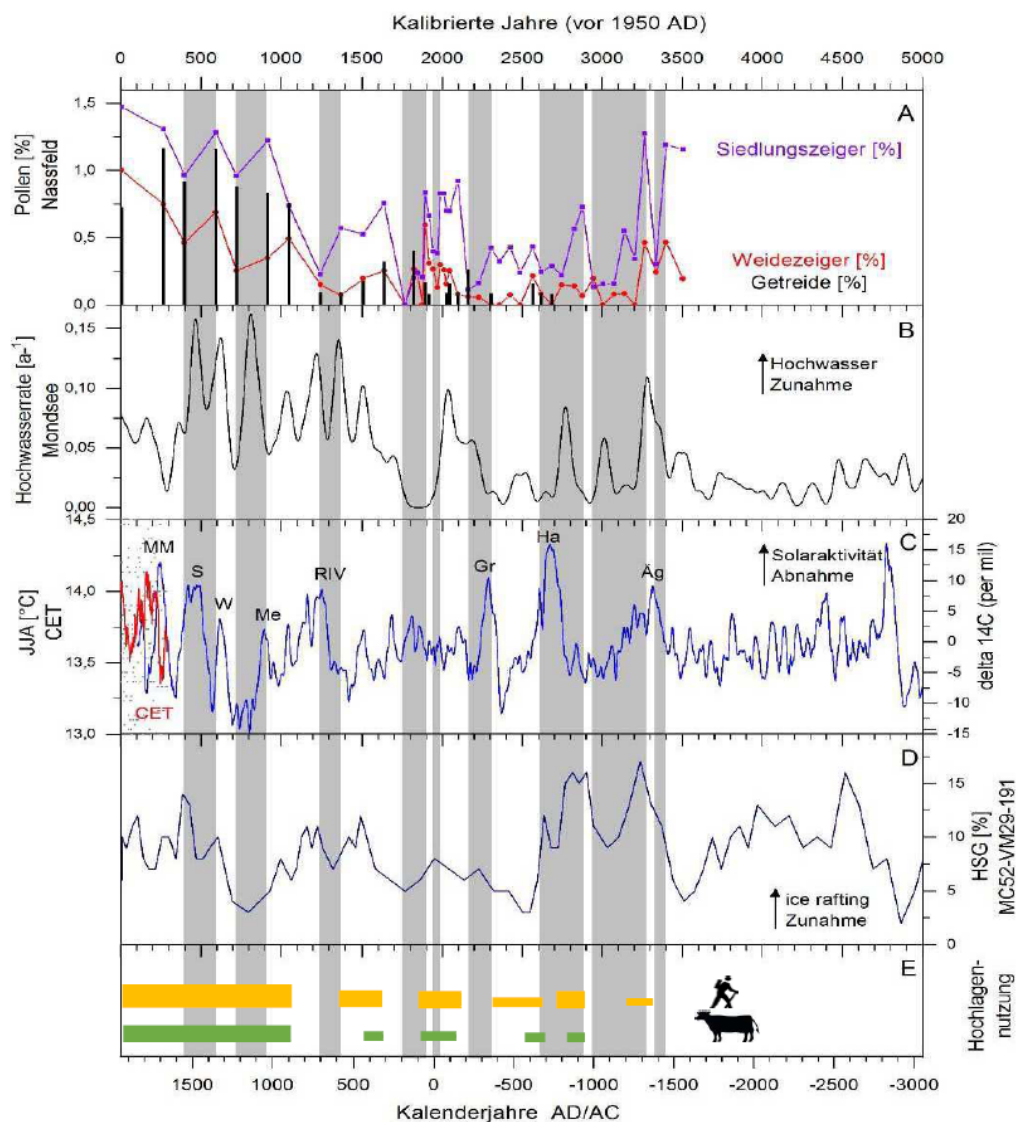
Abbildung 5: Pollenanalytische Untersuchung der A) Siedlungs- und Weidezeiger (%) am Nassfeld (Felber Tauern, Österreich) im Zusammenhang mit der B) Hochwasserrate (a-1) am Mondsee (Swierczynski et al. 2013), C) der Solaraktivität mit C14- Kurve (delta 14 C per mil; Reimer et al. 2004) und Angabe der absoluten Minima: ÄG = ägyptisches Minimum; Ha = Hallstadt Minimum; Gr = Griechisches Minimum; R IV = Römisches IV Minimum; Me = Mittelalterliches Minimum; W = Wolf Minimum; S = Spörer Minimum und MM = Maunder Minimum (Eddy 1976 & 1977; Stuiver & Kra 1986; Stuiver & Braziunas 1988), d) CET (central england temperature; °C), D) der Zu- und Abnahme des ice rafting (HSG %=hematite stained grains, Bond et al. 2001) und E) zeitliche Nutzung der Hochlagen des Felber Tauern; Siedlungszeiger (gelbe Balken); Weidezeiger (grüne Balken). Die grauen längs Balken entlang der Grafik sind eine optische Hilfe zur Erkennung der Zusammenhänge zwischen den einzelnen Parameter.
