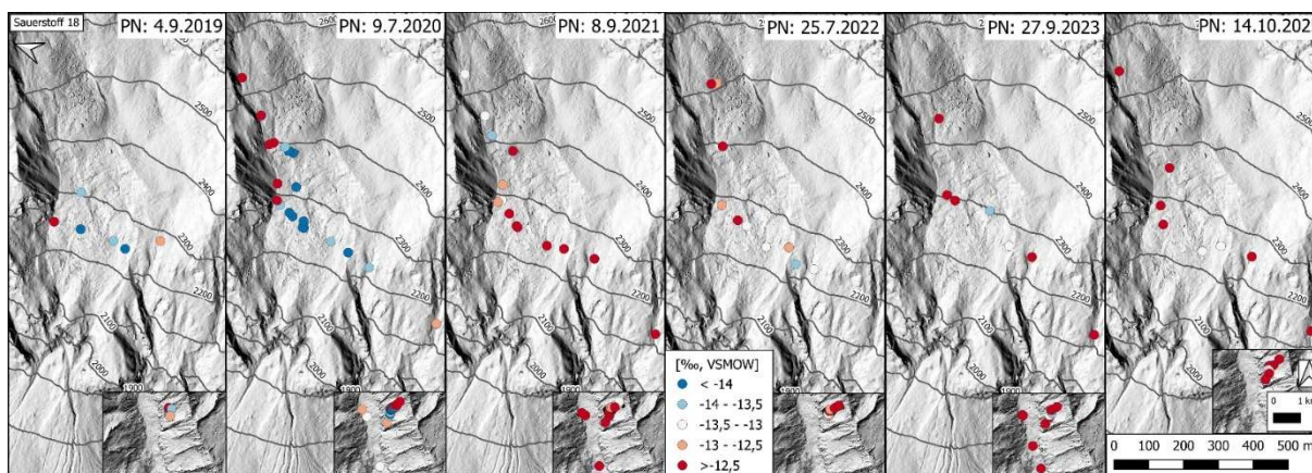
Abbildung 35: Abreicherung von ^{18}\text{O} (Sauerstoff-18) gegenüber VSMOW (Vienna Standard Mean Ocean Water) in den Wasserproben des Sattelkars (2019-2025). Je geringer der Wert, desto weniger schwerer Sauerstoff ( ^{18}\text{O} ) ist in der Probe enthalten und desto „leichter“ ist das Wasser.
