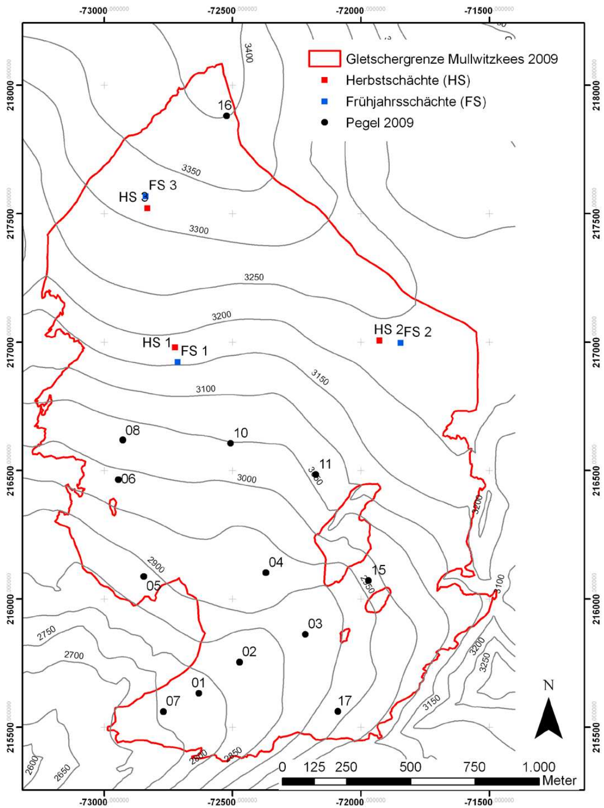
Abbildung 4.1: Mullwitzkees mit Gletschergrenze 2009 (DGPS korrigiert) Lage der Pegel der Frühjahrs- und Herbstschächte.
