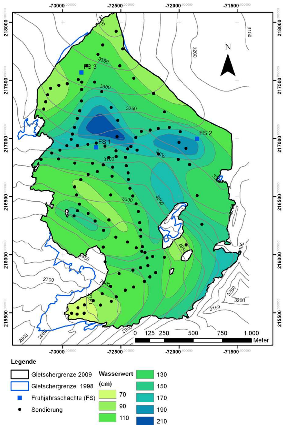
Abbildung 4.2: Flächen gleichen Wasserwertes der Winterbilanz gültig für den 31.05.2010 und Gletschergrenze 1998, sowie Punkte der Sondierungen und Schächte.
