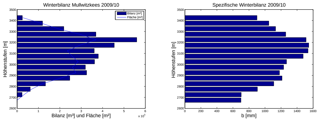
Abbildung 4.3: Nettobilanz [ 10^5 \text{ m}^3 ] und Fläche [ 10^5 \text{ m}^2 ] der Höhenstufen (links) und mittlere spezifische Bilanz [ \text{mm ww} ] der Höhenstufen (rechts) gültig für die Winterbilanz des hydrologischen Jahres 2009/10 am Mullwitzkees.
