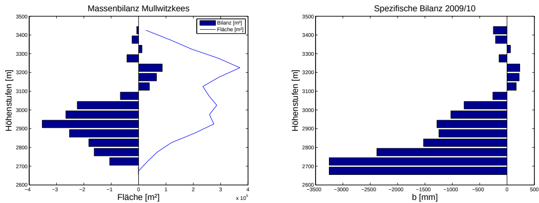
Abbildung 4.5: Nettobilanz [ 10^5 \text{ m}^3 ] und Fläche [ 10^5 \text{ m}^2 ] der Höhenstufen (links) und mittlere spezifische Bilanz [ \text{mm ww} ] der Höhenstufen (rechts) gültig für die Jahresbilanz des hydrologischen Jahres 2009/10 am Mullwitzkees.
